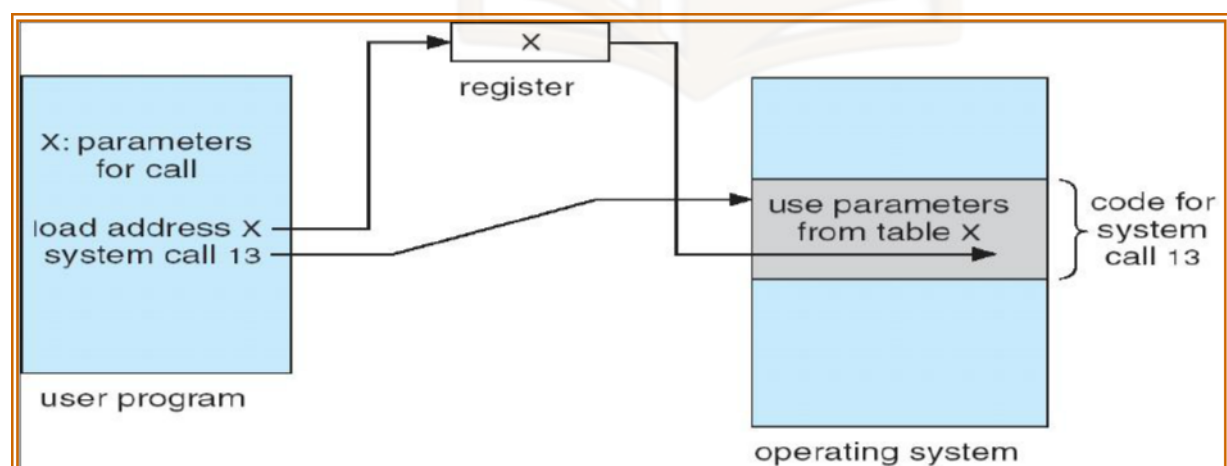
Figure 15: Parameter passing via table
